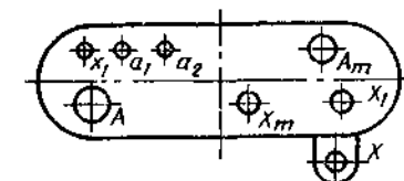
а) автотрансформатор АОДЦТН-333000/750/330
